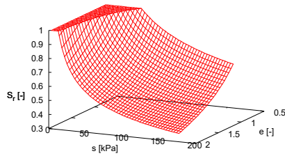
Mašín (2010)
