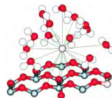
Ion-Dipole
